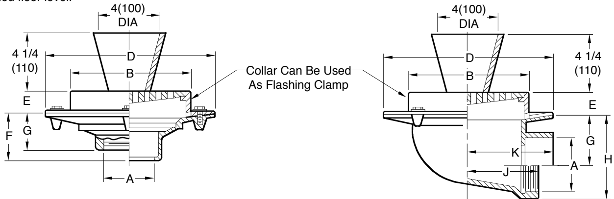
8 1/2"(215) 12"(305) . . . TOP SIZE = B DIA . . . . . 8 1/2"(215) 12"(305) Fig. . . . 3710C . . . 3715C . . . CAULK OUTLET . . . . . Fig. . . . 3720C . . . 3725C Fig. . . . 3710T . . . 3715T . . . THREADED OUTLET . . . Fig. . . . 3720T . . . 3725T
